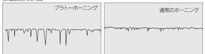
断面曲線模式図
