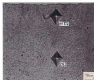
低圧浸炭層の顕微鏡組織
