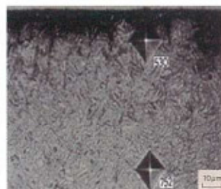
Rxガス浸炭層の顕微鏡組織
